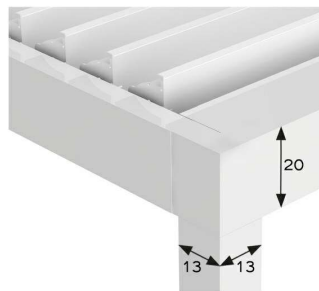
PARTICOLARE ANGOLO
