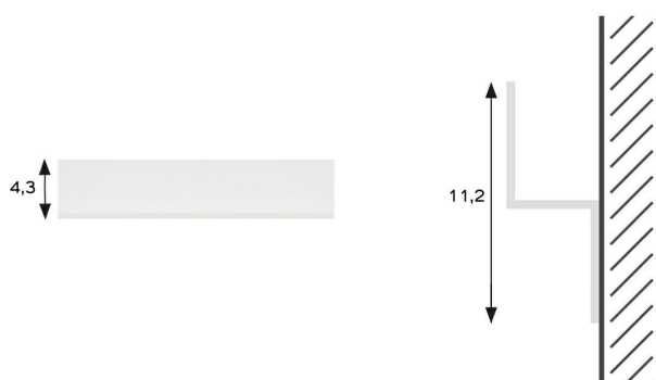
STAFFA A PARETE Frangisole
