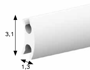
RINFORZO ③
