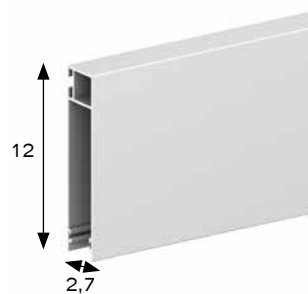
GUIDA ②
