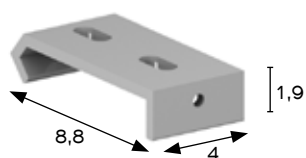
PIASTRA IN ALLUMINIO A SCOMPARSA
