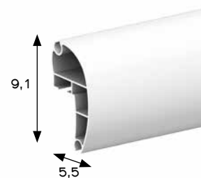
TERMINALE ⑤
