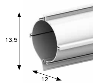
CASSONETTO ②
