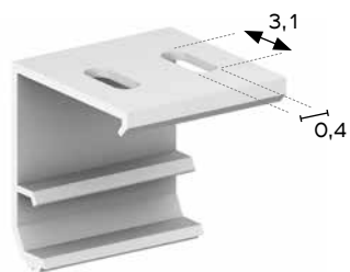
PIASTRA ATTACCO SOFFITTO
