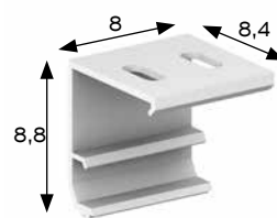
PIASTRA ①
