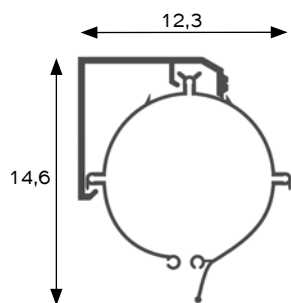
ATTACCO PARETE
